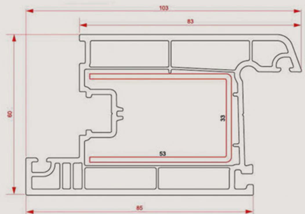
60 mm Kapi Kanat Profili 60 mm Door Sash Profile
