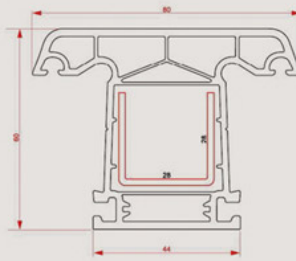
60 mm Orta Kayıt Profili 4 Odacıklı 60 mm Mullion Profile W / 4 Chamber
