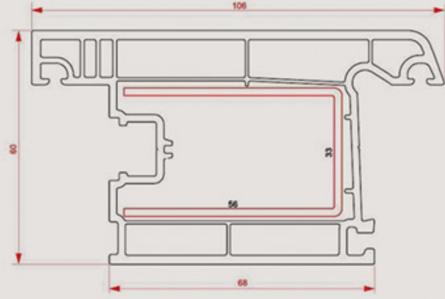
60 mm Dışa Açılır Kapi Kanat Profili 60 mm Outside Opening Door Sash Profile
