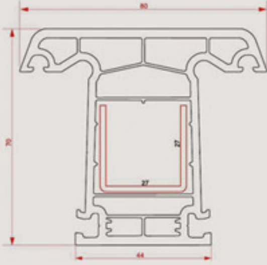
70 mm Orta Kayıt Profili 5 Odacıklı 70 mm Mullion Profile W / 5 Chamber
