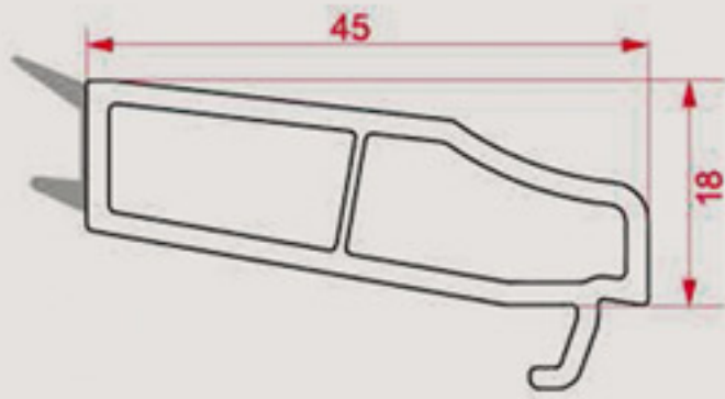
4 mm 70'lik Çıta 4 mm 70' Bead
